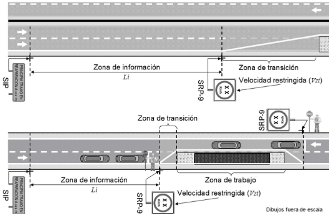
FIGURA 7.- Señales verticales que indican el principio y fin de la zona de información ( L_i )
